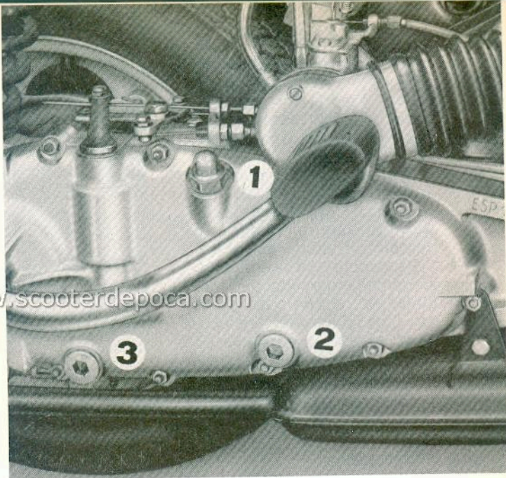
1. Tappo di carico - 2. Tappo di livello - 3. Tappo di scarico.
